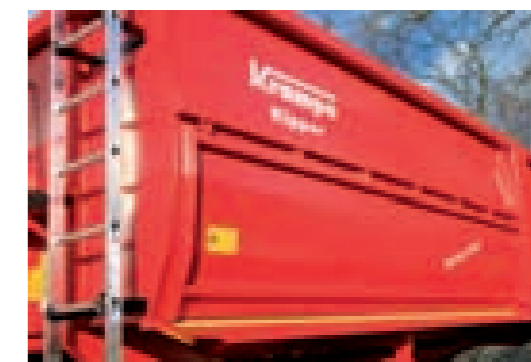
Die seitlichen Bordwände werden auf ganzer Länge mit einer Anpresslippe korndicht abgedichtet. Der alte Schließhaken hat bei uns schon lange ausgedient.
