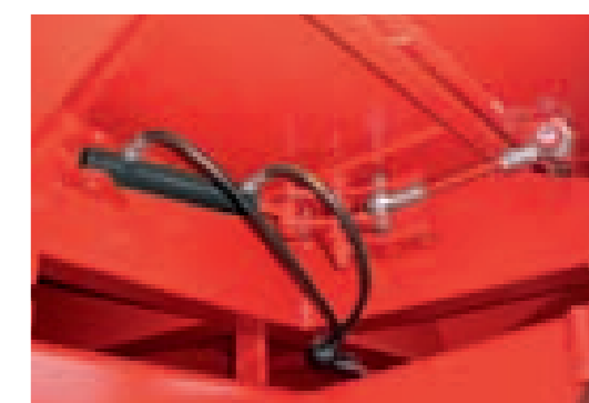
Die hydraulische Entriegelung der seitlichen Bordwände kann bequem vom Schleppersitz aus erfolgen. Der Übertotpunkt-Verschluss sichert gegen unbeabsichtigtes Öffnen.
