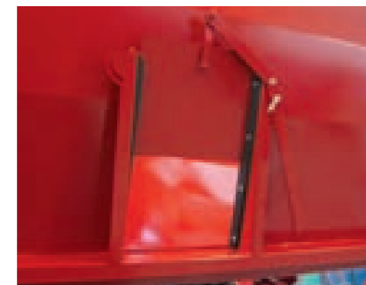
Alle Wannenkipper haben einen leichtgängigen Auslaufschieber (46x34 cm), der in Kunststoffführungen läuft. Der Öffnungshebel ist wahlweise rechts oder links montierbar.
